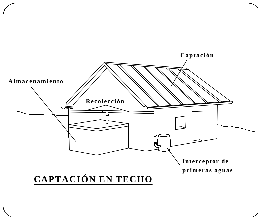
Figura 1. SCAPT - SISTEMA DE CAPTACION DE AGUA PLUVIAL EN TECHOS
